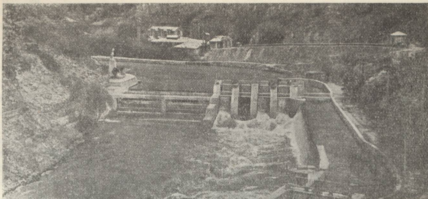
Уже десять лет работает Канакирская гидроэлектростанция. Она даёт свет ближайшим городам и колхозам.
